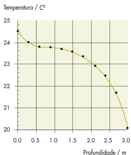
Figura 6 - Perfil de temperatura medido na corta da Mina de São Domingos. A medição foi efectuada cerca das 13h, tendo durado cerca de 30m.
